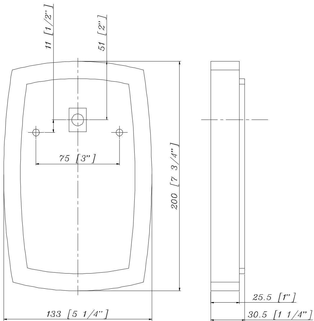
3153/3154壁板
